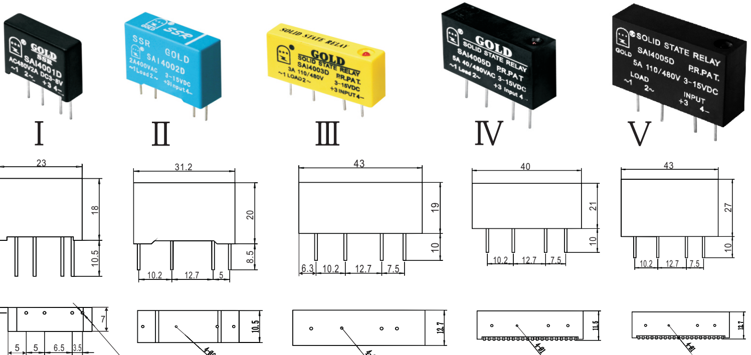
外形尺寸: mm
