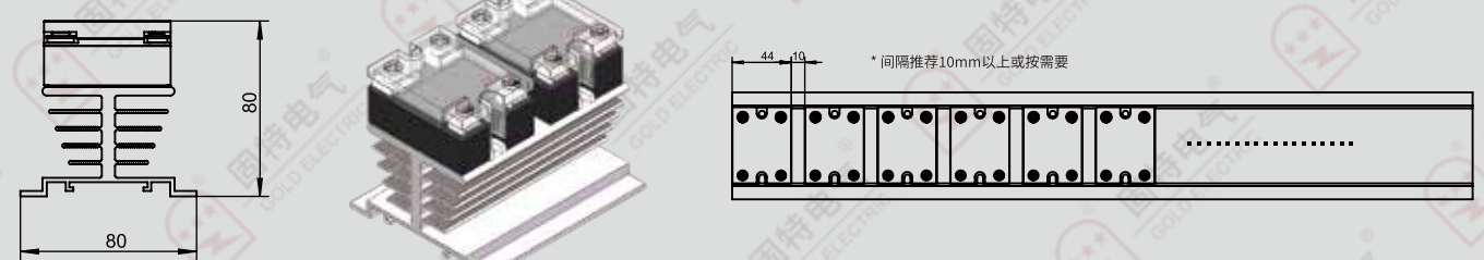
X型散热器 额定电流5-10A, 推荐选用X型散热器
