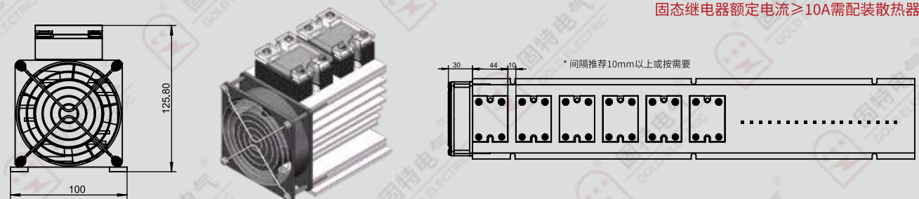
T型散热器 额定电流 \geq 30\text{A} , 推荐选用T型散热器
