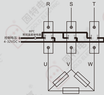
负载三角型接线示意图
